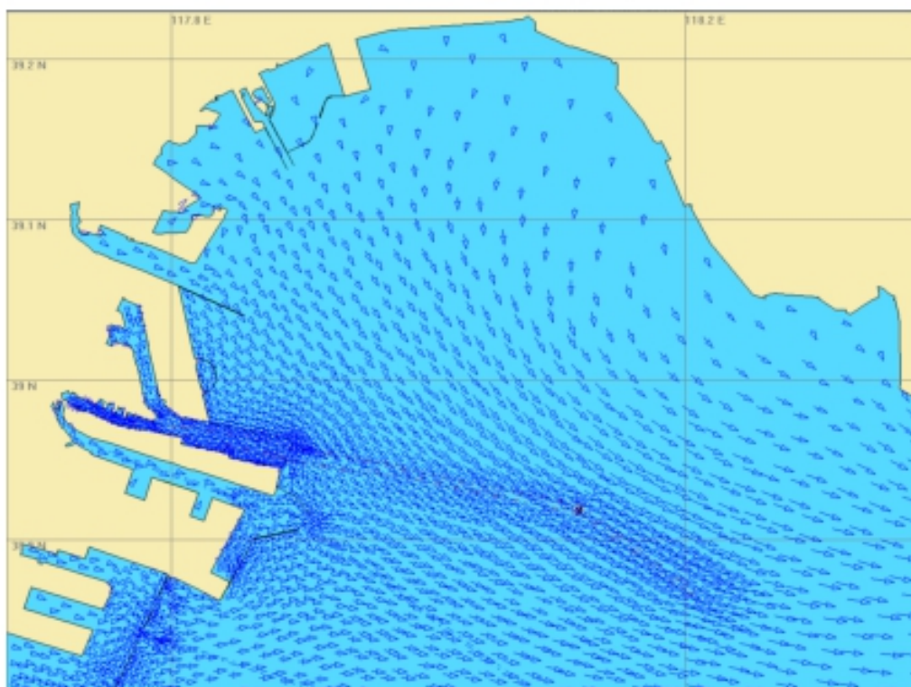
图 4-3-5 大范围潮流场（落潮阶段）示意图
