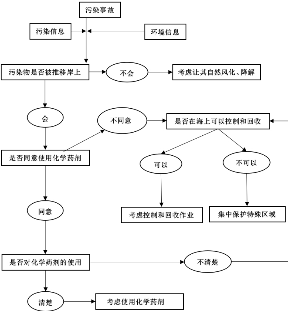
图 7-5-1 海上溢油污染事故应急决策流程示意图
