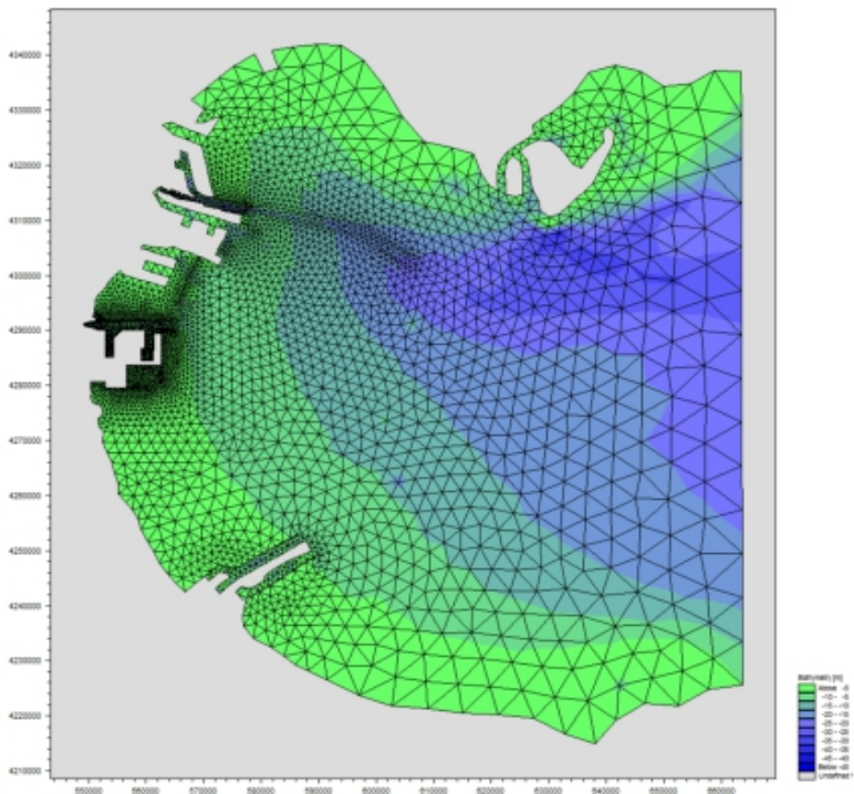
图 4-3-3 计算范围及网格剖分示意图
